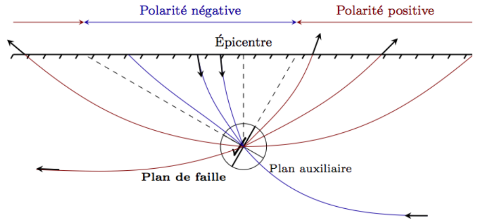
Schéma 2D du foyer sismique et des quadrants compressifs et extensifs.
