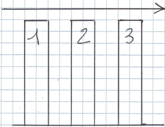
amortissement linéaire
