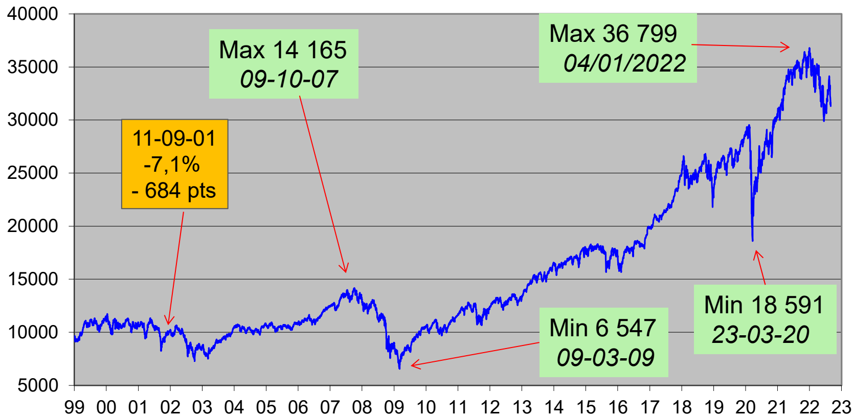
DJIA du 04 janvier 1999 à actuel (en Close quotidien)
