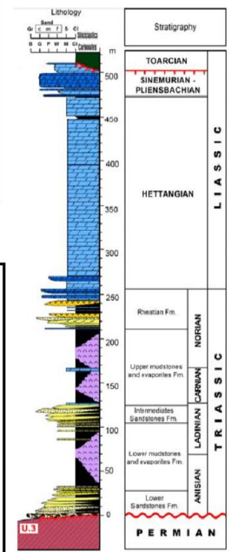
Log lithologique des environs de Pégairolle de l'Escalette
