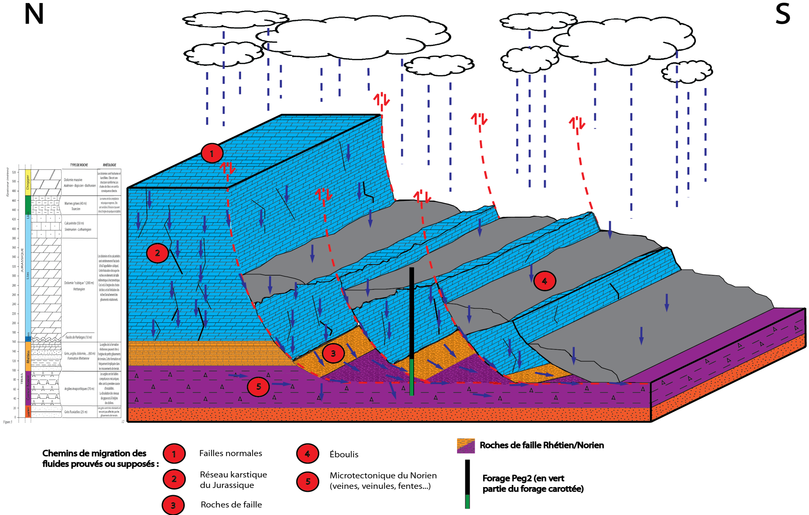
Figure 40 : Chemins de migration prouvés ou supposés avec leurs lithologies associées (source : Giovannangeli Nicolas) + Log lithologique de la zone (source : d'après M. LOPEZ, non publié).
